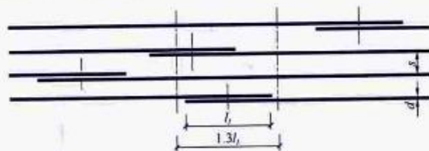
图1 钢筋绑扎搭接接头连接区段及接头面积百分率
